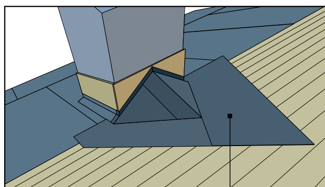
подкладочный ковер Рис. 51
