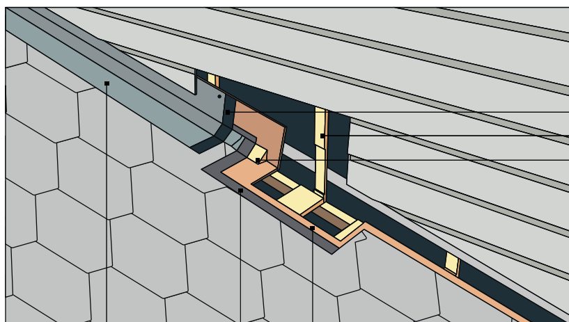
Ендовый ковер Рис. 69 Подкладочный ковер OSB
