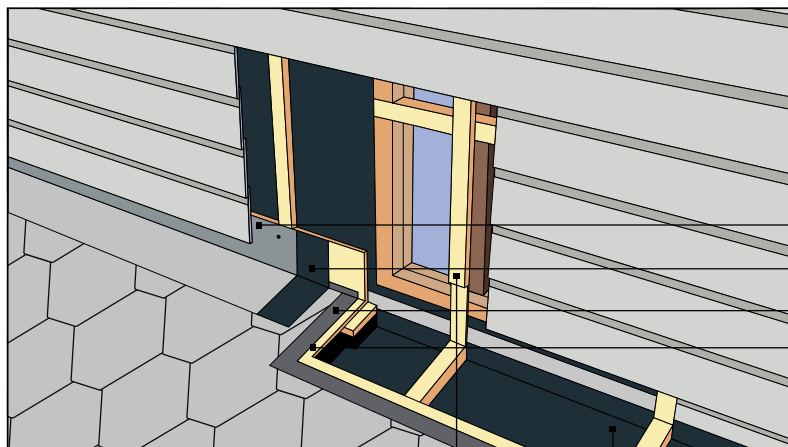
Обрешетка Фасада Рис. 68 Гидроизоляция
