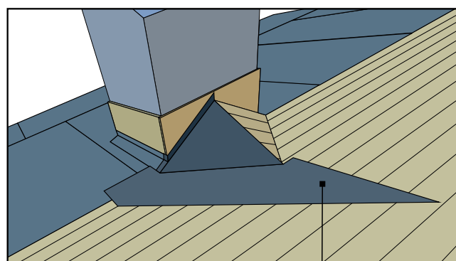
подкладочный ковер Рис. 50
